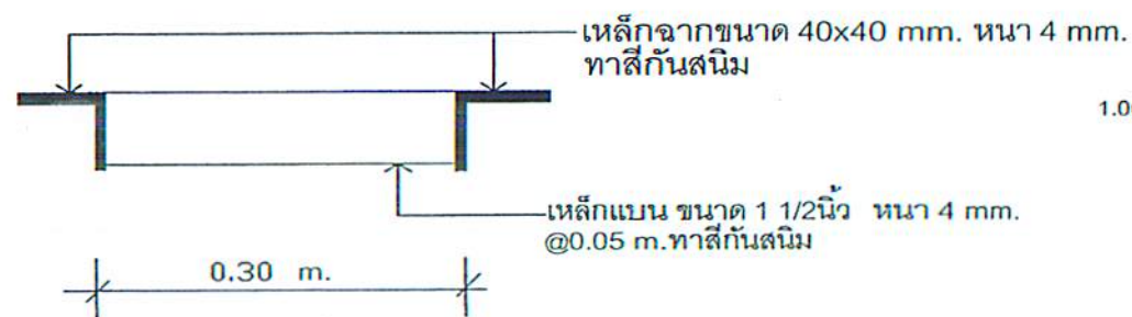
รูปตัดแสดงฝาเหล็กปิดร่องระบายน้ำ
