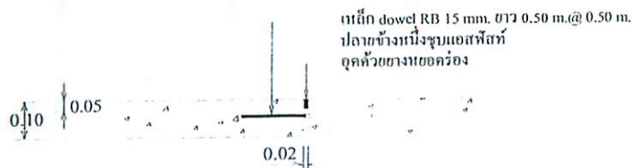
แบบขยาย(3) CONSTRUCTION JOINT Scale 1:25
