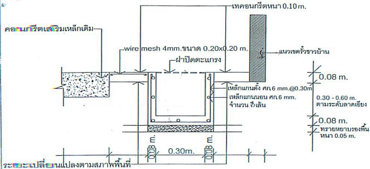
รูปตัด ก-ก
