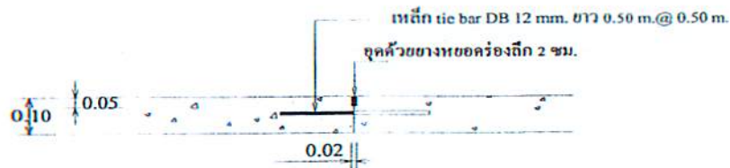
แบบขยาย(2) LONGITDINAL JOINT Scale 1:25
