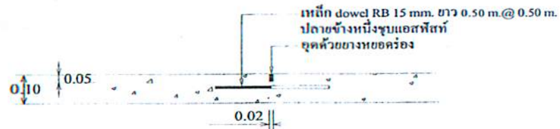
แบบขยาย(3) CONSTRUCTION JOINT Scale 1:25
