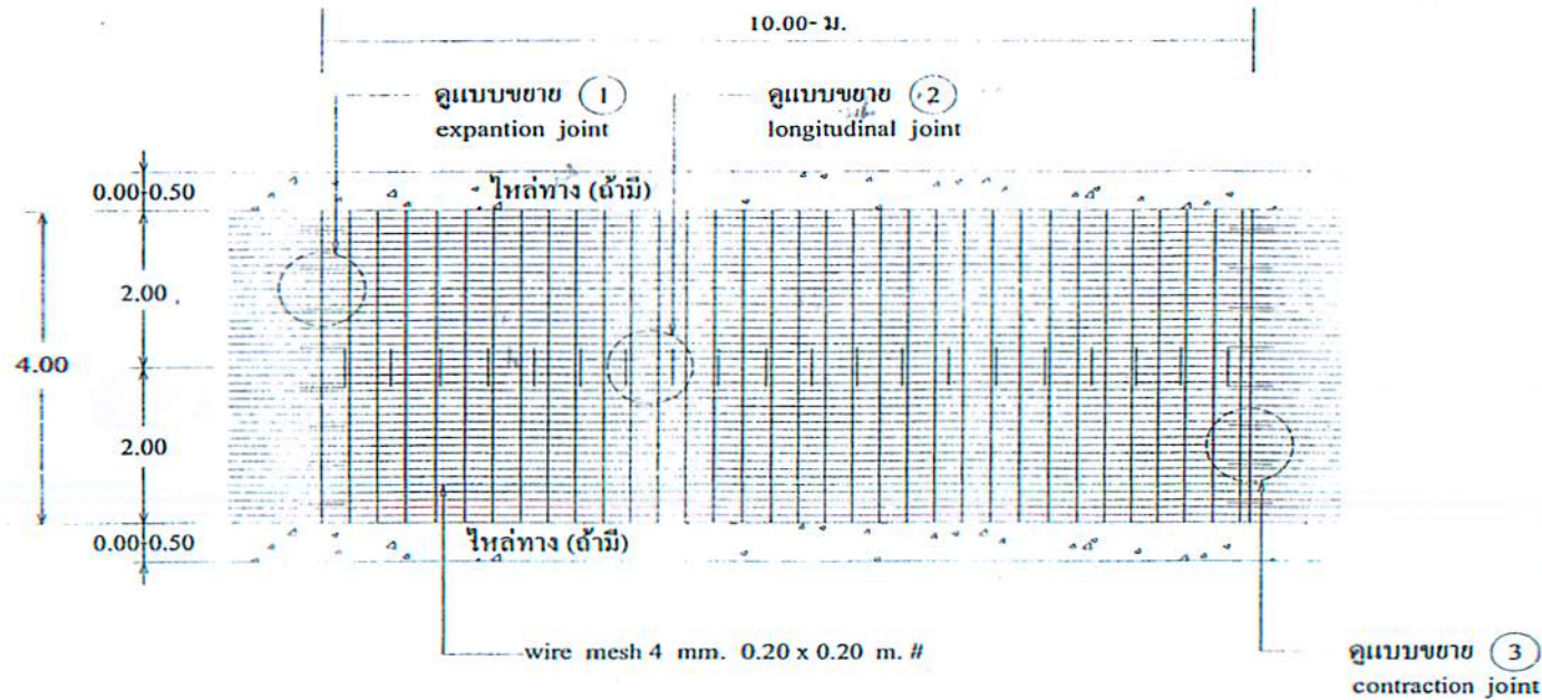
แปลนการวางตะแกรงเหล็ก
